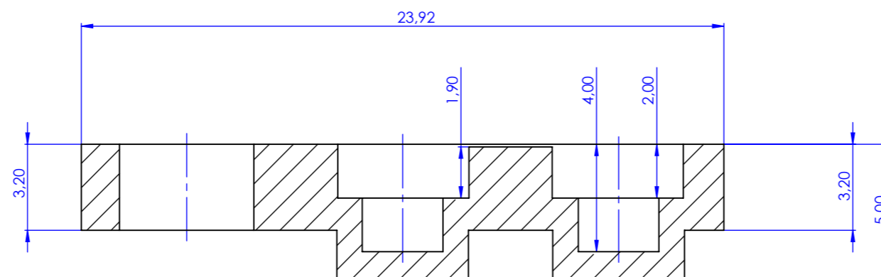
PRZEKRÓJ A-A
