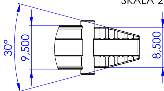
SZCZEGÓŁ E SKALA 2 : 1
