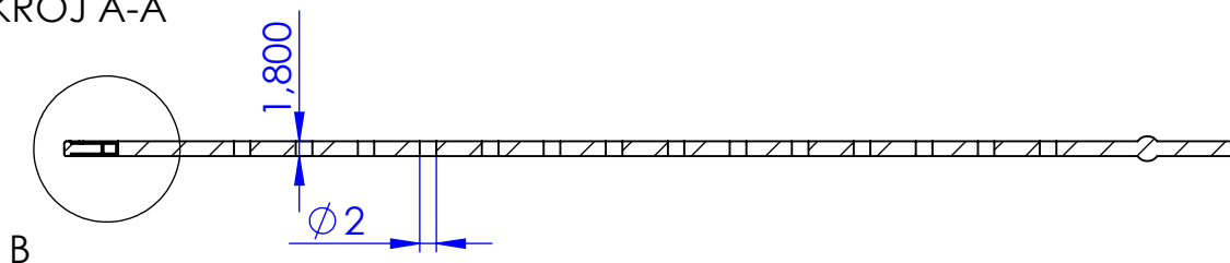
PRZEKRÓJ A-A
