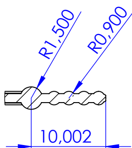
SZCZEGÓŁ D SKALA 2 : 1
