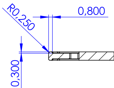
SZCZEGÓŁ B SKALA 2 : 1
